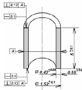
Cilindru fără guler
